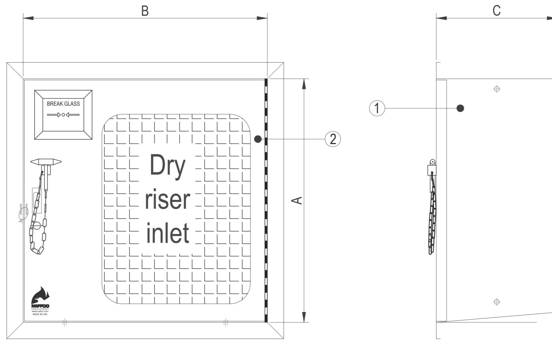
ELEVATION
